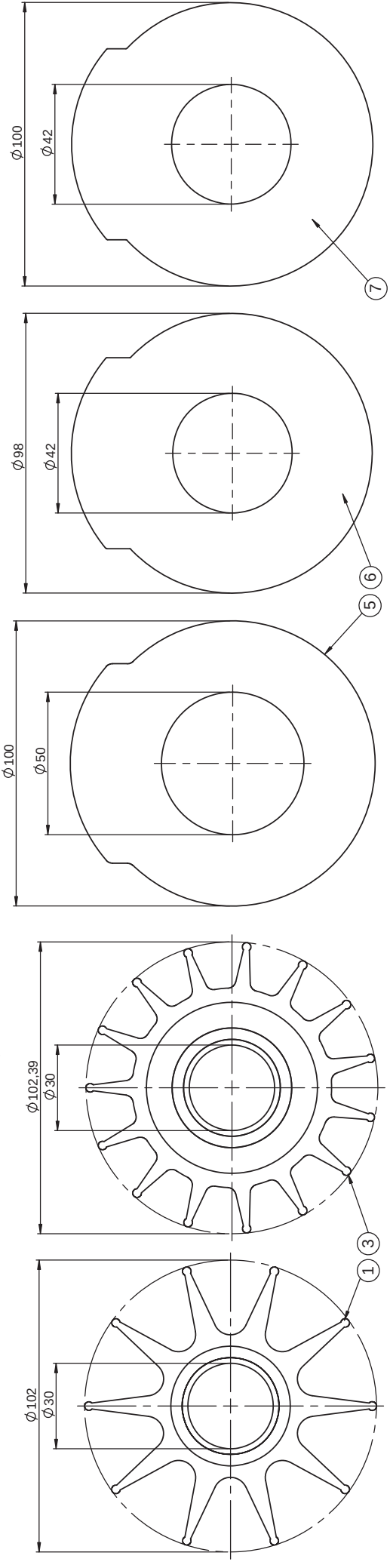
Zellenräder / Cellular wheels / Roues de distribution
